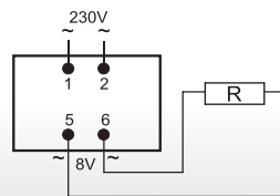
Schéma zapojení
