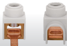
Připojení do přístrojů pomocí konektoru kolík (jazýček)
